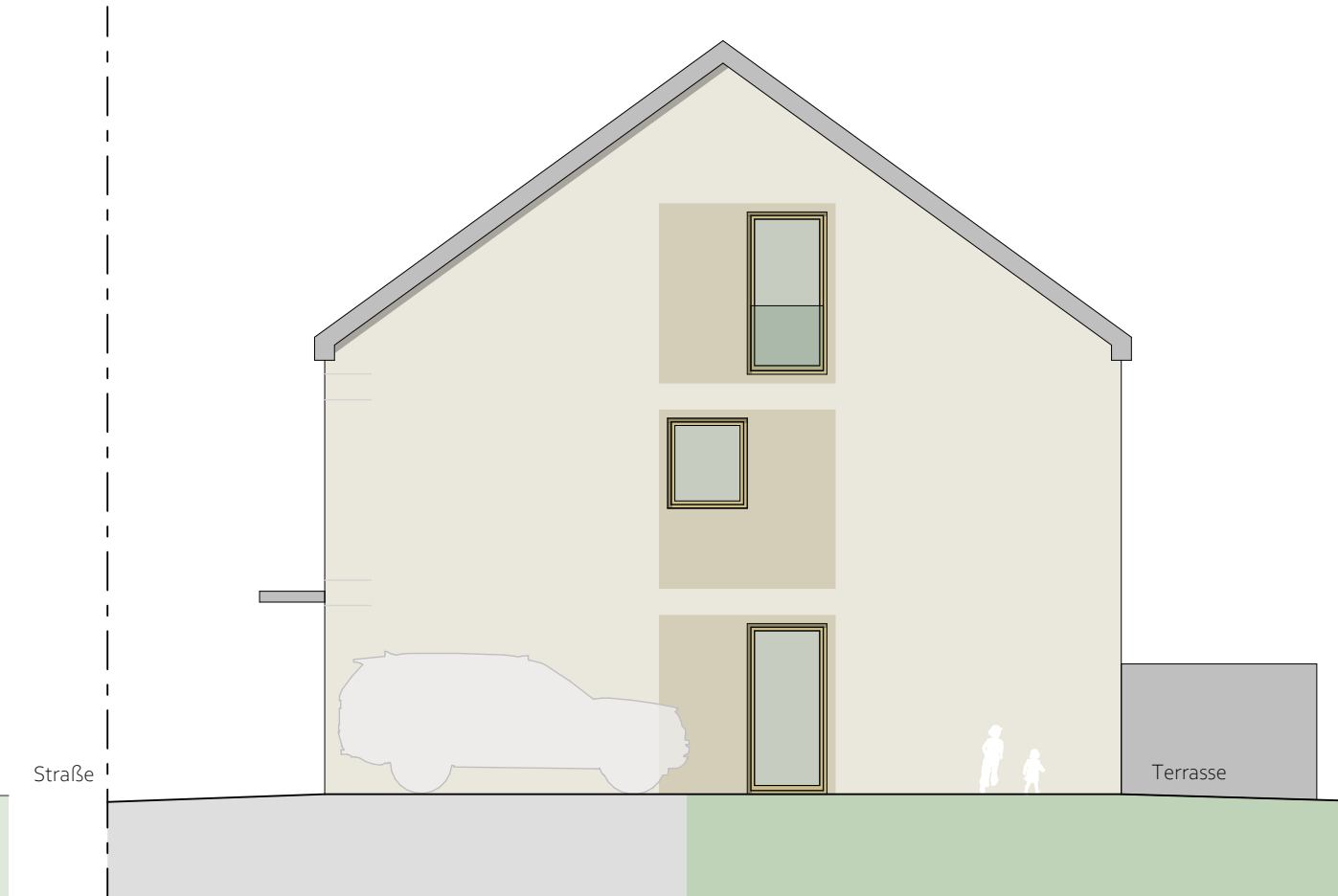
Giebelansicht O/W
